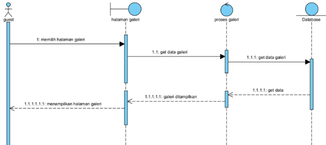
Gambar 9 Sequence Diagram Melihat galeri
