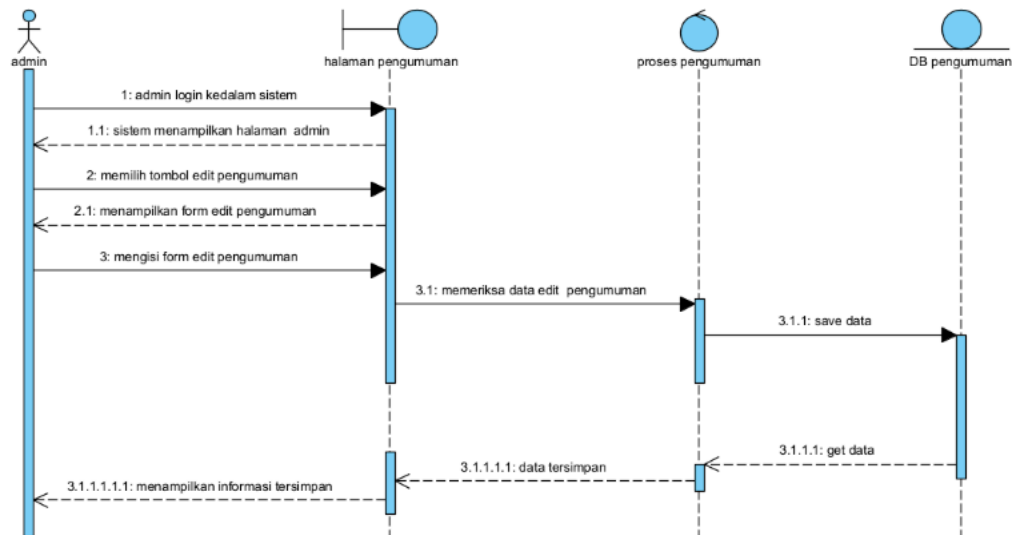
Gambar 34 Sequence Diagram mengedit pengumuman
