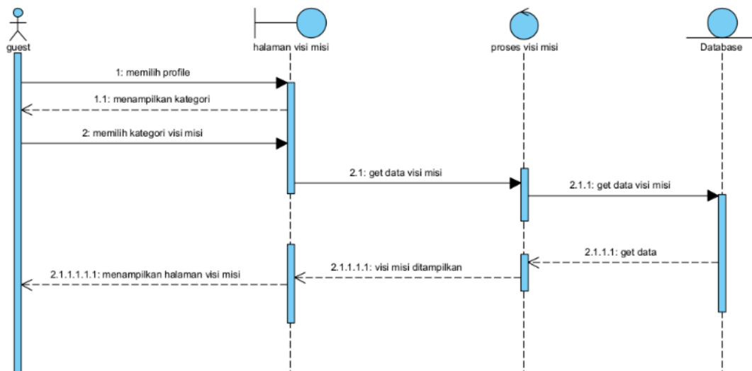
Gambar 6 Sequence Diagram Melihat visi misi
