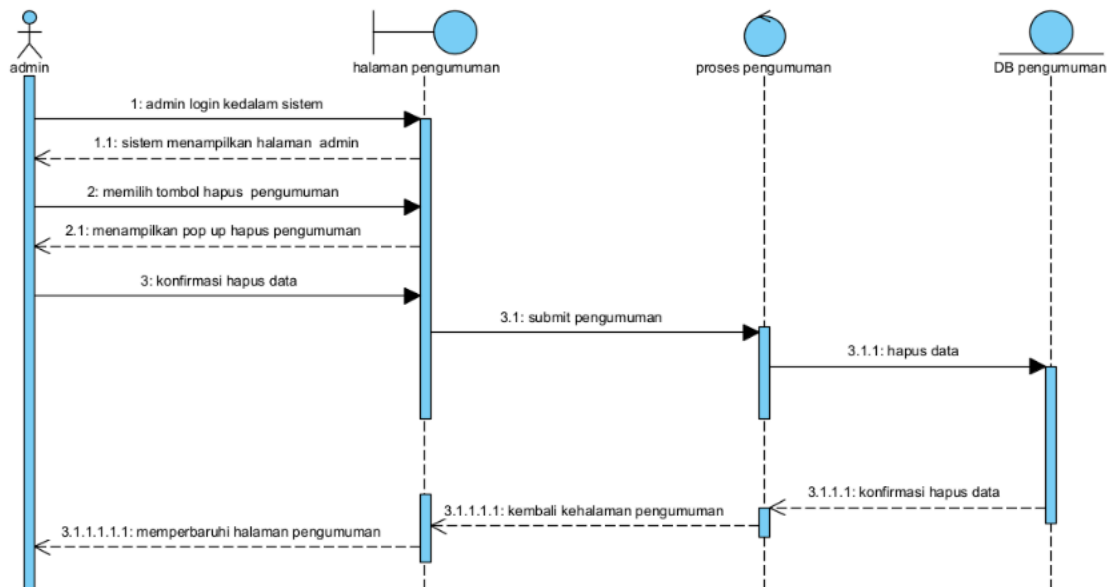
Gambar 31 Sequence Diagram menghapus pengumuman
