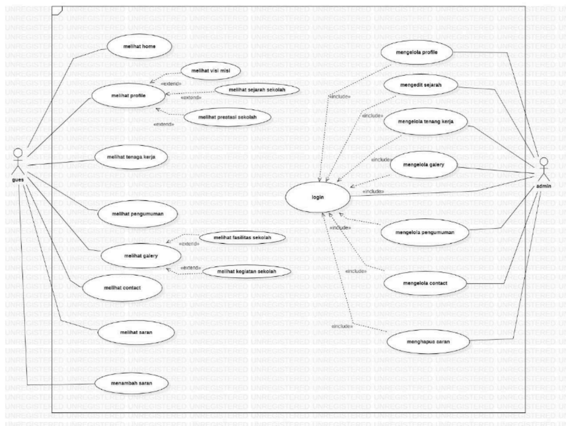
Gambar 2 Use Case Diagram SD Negeri 173551 Laguboti
