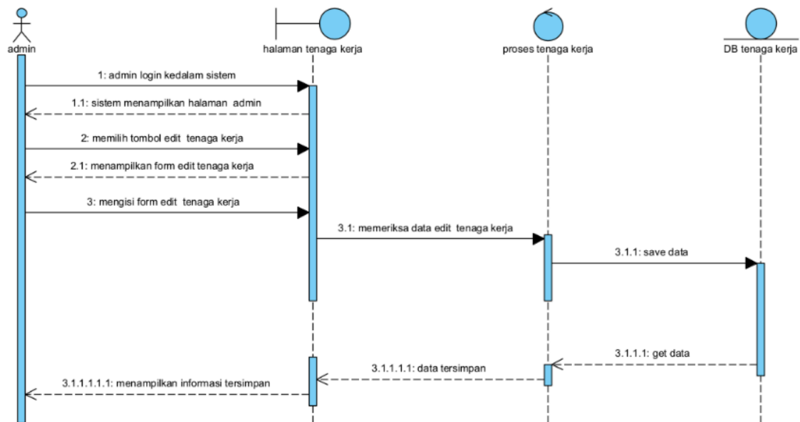
Gambar 21 Sequence Diagram mengedit tenaga kerja
