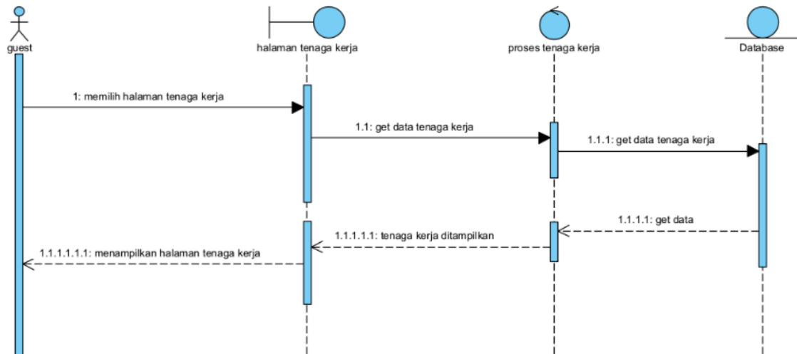
Gambar 11 Sequence Diagram Melihat tenaga kerja
