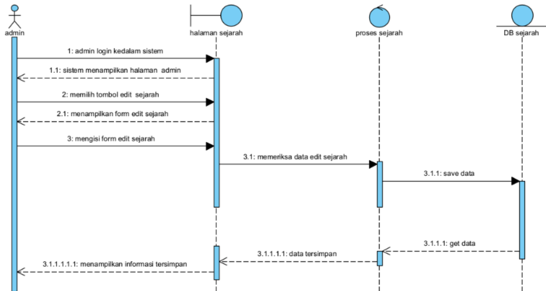
Gambar 24 Sequence Diagram mengedit sejarah
