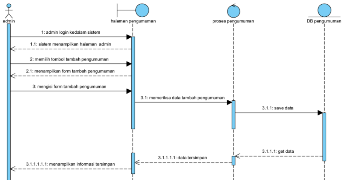
Gambar 17 Sequence Diagram menambah pengumuman
