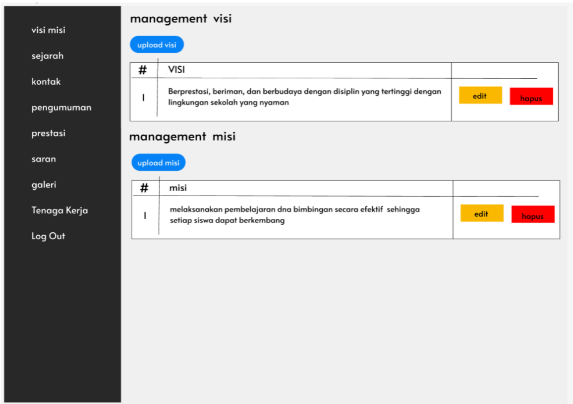
Gambar 48 Halaman Menghapus Visi Misi Pada Admin
