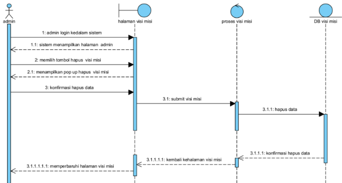
Gambar 27 Sequence menghapus visi misi
