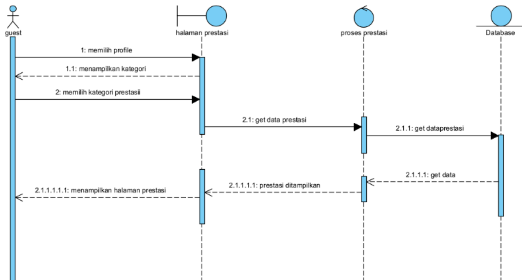
Gambar 7 Sequence Diagram Melihat prestasi
